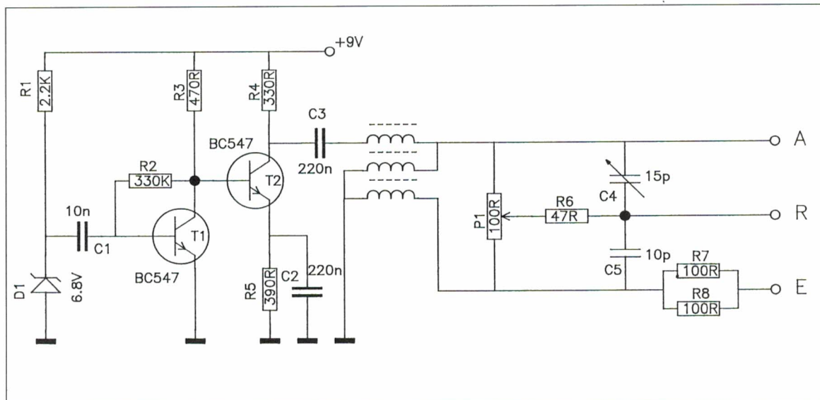
Fig 6 Schema ruisbrug
