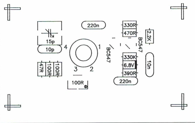
Fig 9 Componentenopstelling ruisbrug
