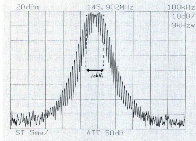
Figuur 1 Maximale frequentie-zwaai zender FM-modulatie
