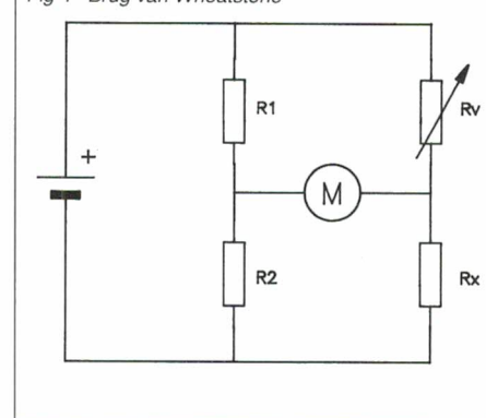
Fig 4 Brug van Wheatstone
