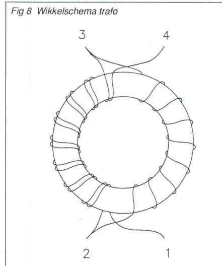
Fig 8 Wikkelschema trafo
