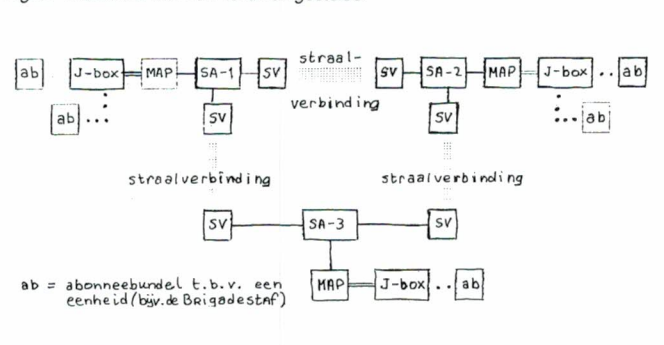
Fig. 2 Voorbeeld van een verbindingstelsel
