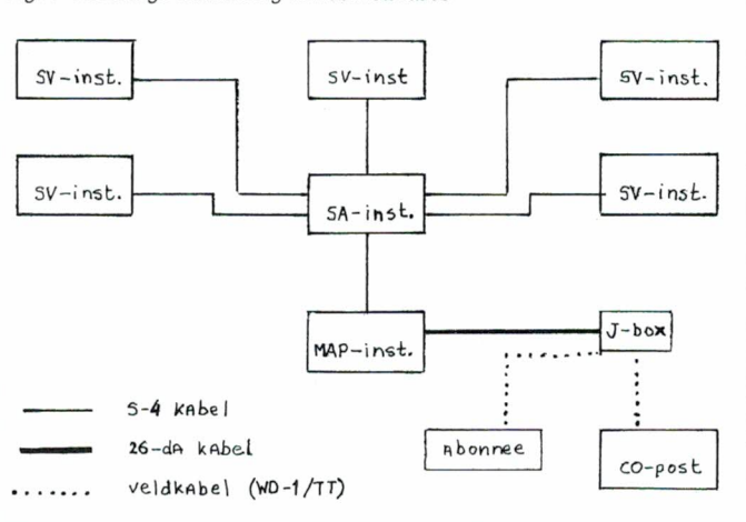
Fig. 1 Onderlinge samenhang van de installaties
