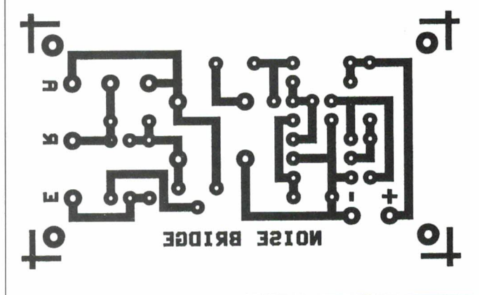
Fig 10 Koperzijde ruisbrug
