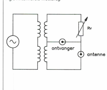
Fig 5 Antennenuis-meetbrug
