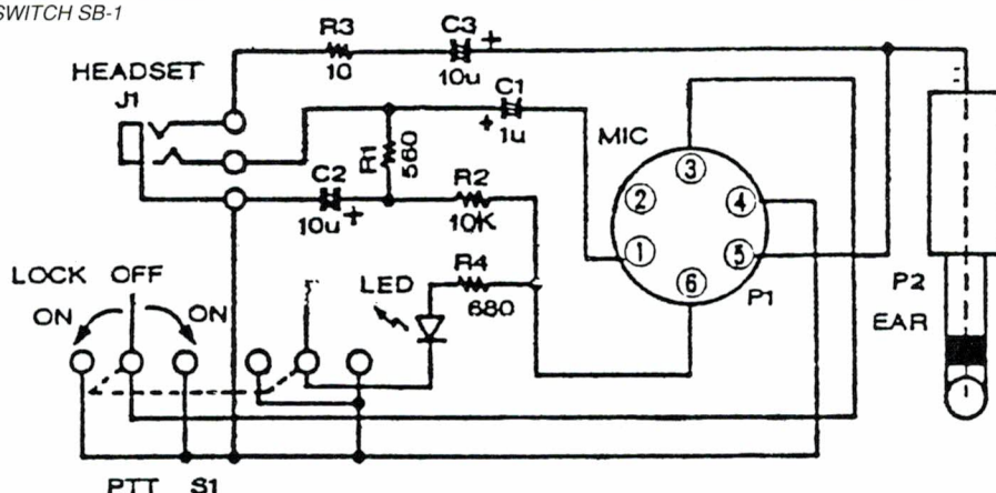
PTT SWITCH SB-1
